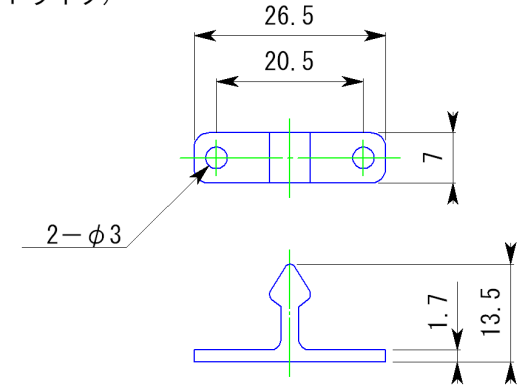
受板(ストライク)
