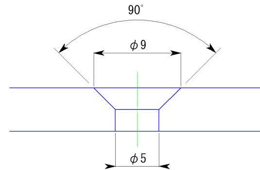
皿モミ部拡大図
