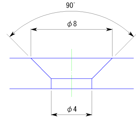
皿モミ部拡大図
