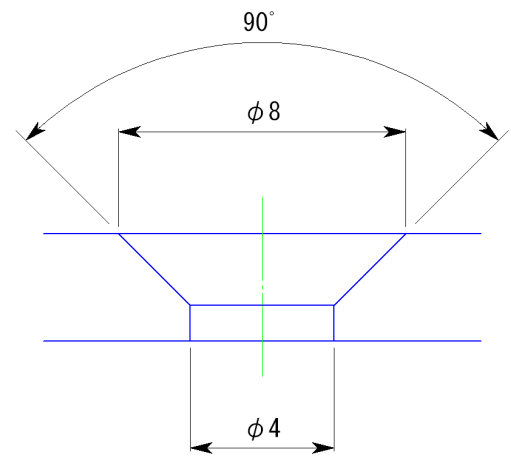
皿モミ部拡大図
