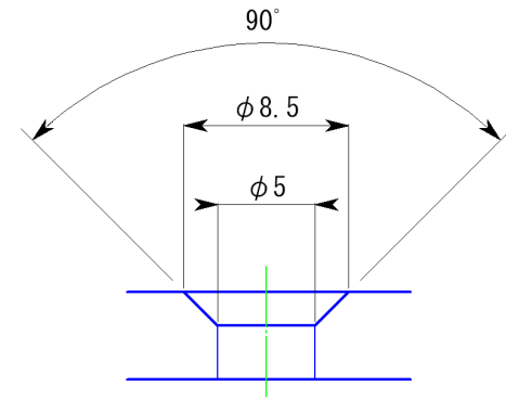
皿モミ部拡大図
