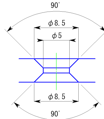
皿モミ部拡大図
