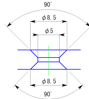
皿モミ部拡大図
