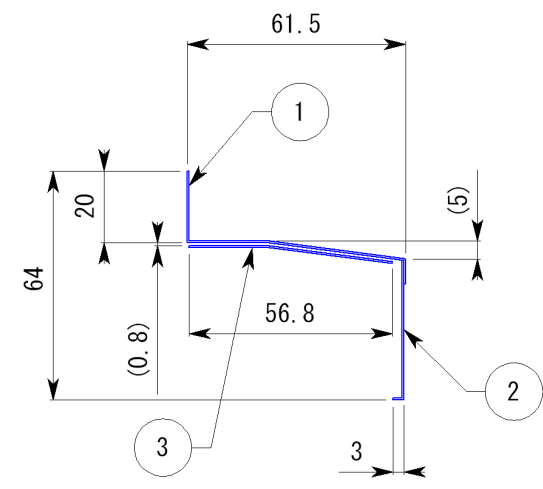
A-A' 断面図
