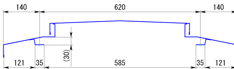
ブラケット部断面図
