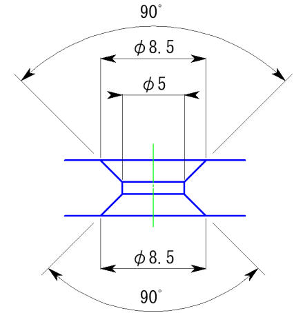
皿モミ部拡大図
