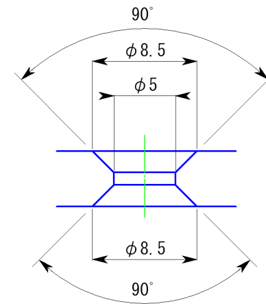
皿モミ部拡大図
