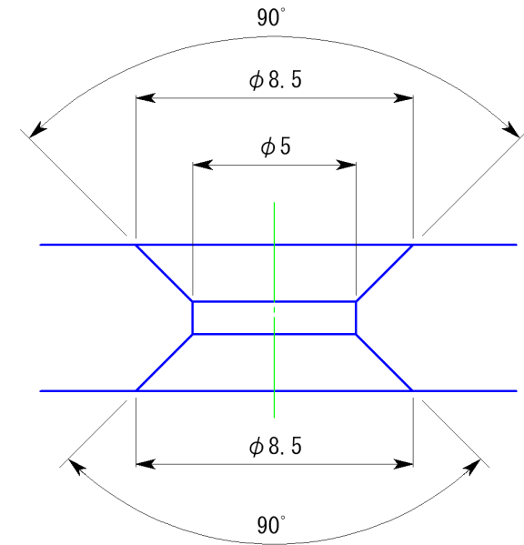
皿モミ部拡大図
