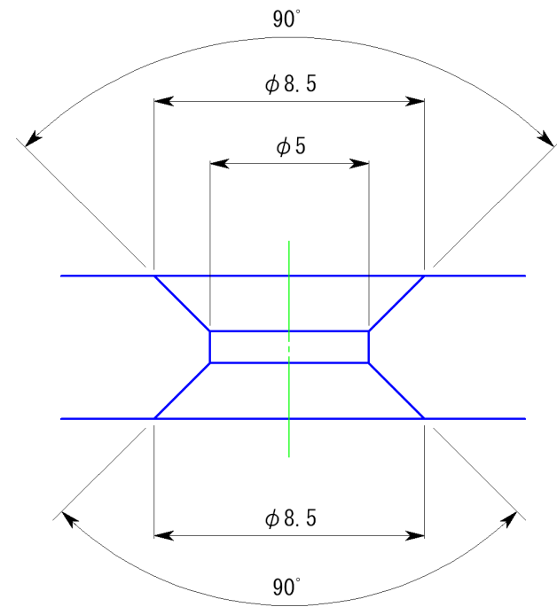
皿モミ部拡大図
