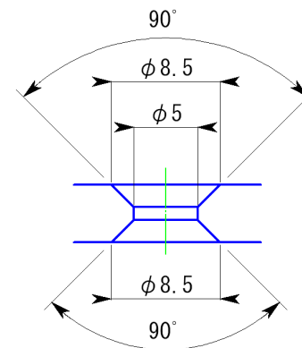
皿モミ部拡大図
