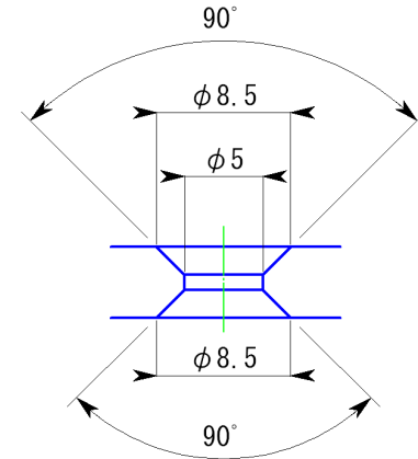
皿モミ部拡大図
